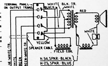
Fig. 2—Speaker Wiring
